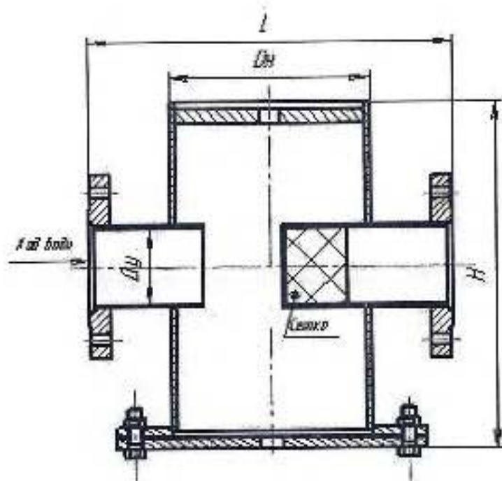
2 Исполнение фланцевое
